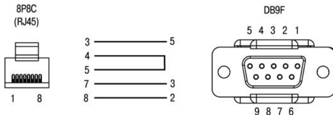
Рисунок Г.1 – Схема кабеля программирования КС14, входящего в комплект поставки
