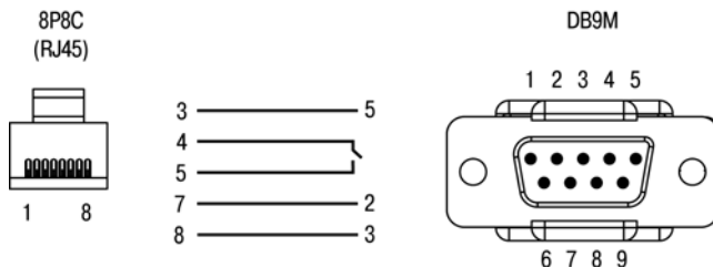
Рисунок Г.3 – Схема кабеля KC17 «ПЛК–Модем»
