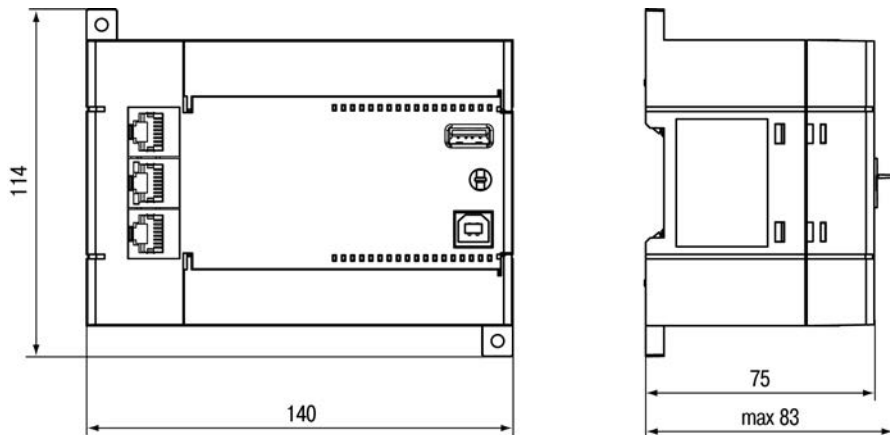
Рисунок А.2 – Габаритные размеры ПЛК110.X.32.X-X(M02) и ПЛК110.X.30.X-X(M02)
