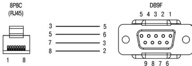
Рисунок Г.2 – Схема кабеля КС16
